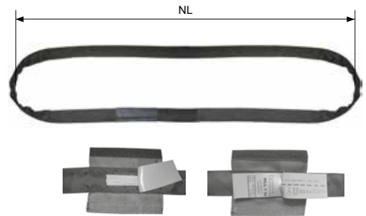
Sichtfenster zur Kontrolle der Drahtseileinlage mit verschließbaren Schutzklappen. Verdecktes Kennzeichnungsetikett.
