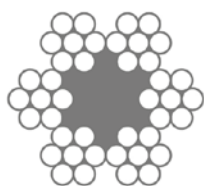
Abspannseil
