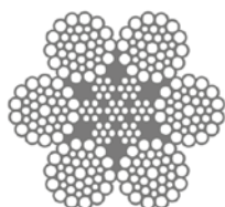
Schrappenseil, Windenseil
